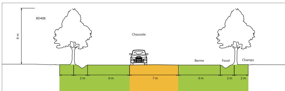
Coupe transversale de l'alignement de platanes sur la RD 408
